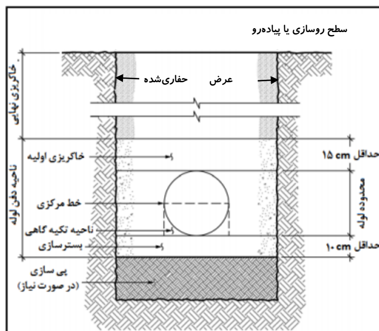
شکل ۳۶: مقطع عمومی ترانشه های لوله‌ها
