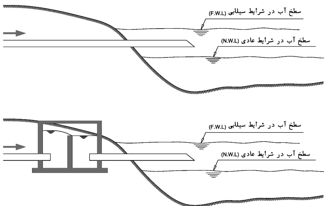
شکل ۳۰: تخلیه ثقلی به آب‌های پذیرنده
