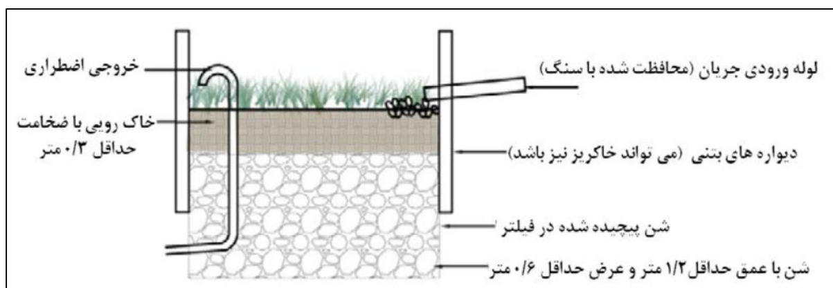
شکل ۱۰: نمایی از یک حوضچه نفوذی زیستی
