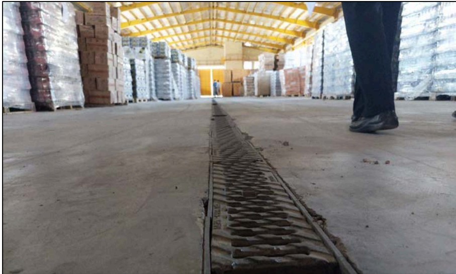
شکل ۱۵: استفاده از کانال پیش‌ساخته مشبک (trench Drain) در سوله انبارها
