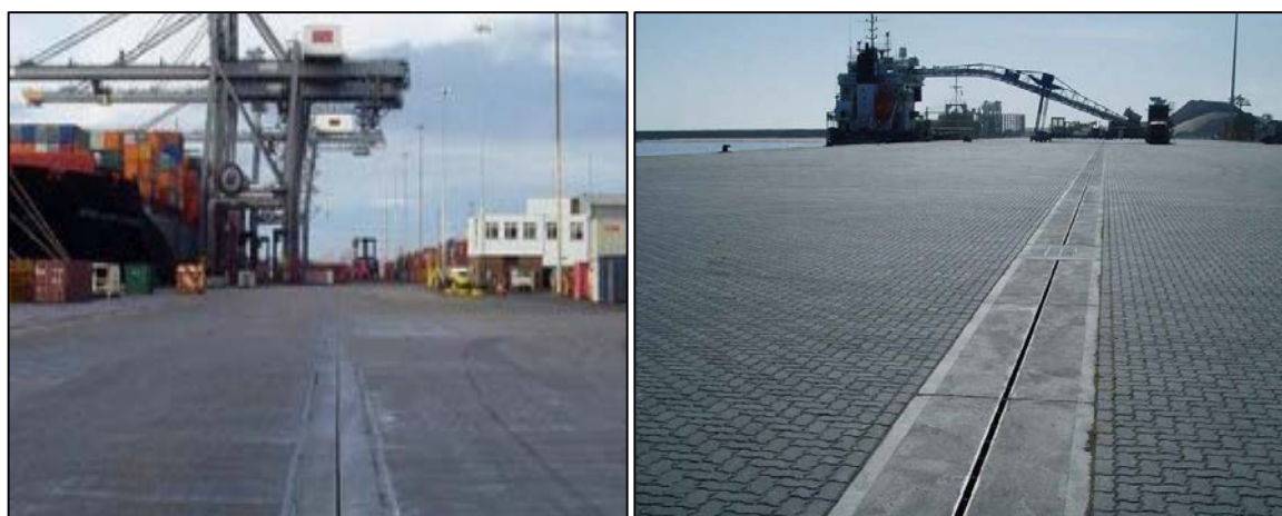
شکل ۵: نمونه ای از سیستم زهکشی سطحی با کانال پیش ساخته خطی
