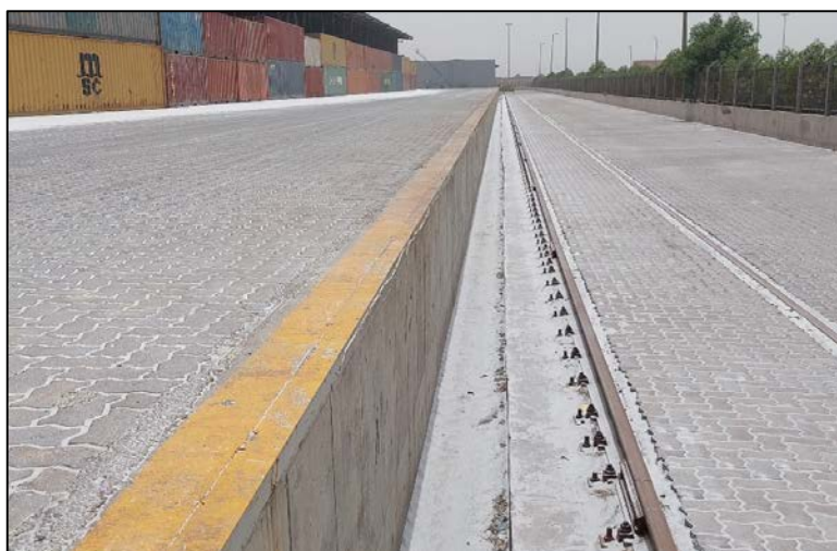
شکل ۱۶: کانال روباز مجاور خطوط ریل برای زهکشی محوطه ریلی
