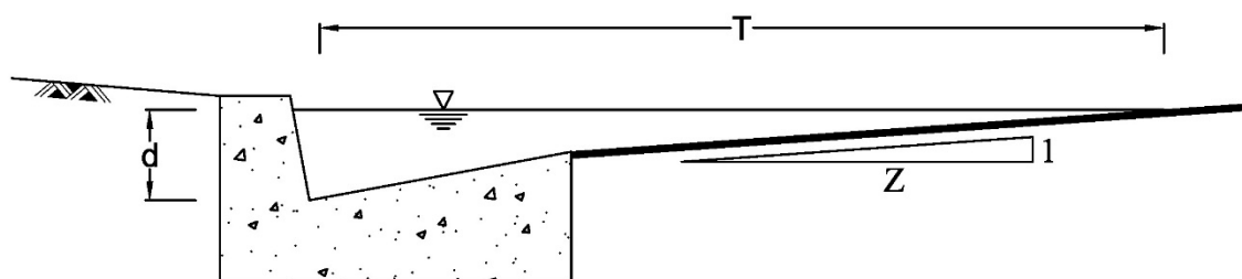
شکل ۲۳: مقطع عرضی کانپو
