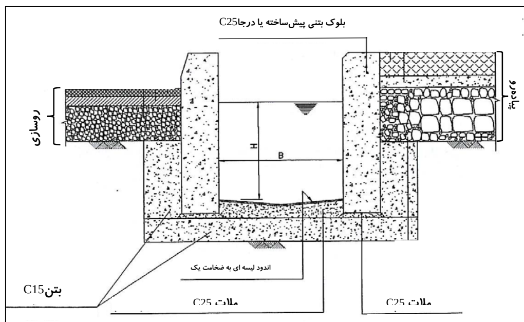
شکل ۳۳: جزییات عمومی اجرای کانال روباز (پیش‌ساخته و درجا)
