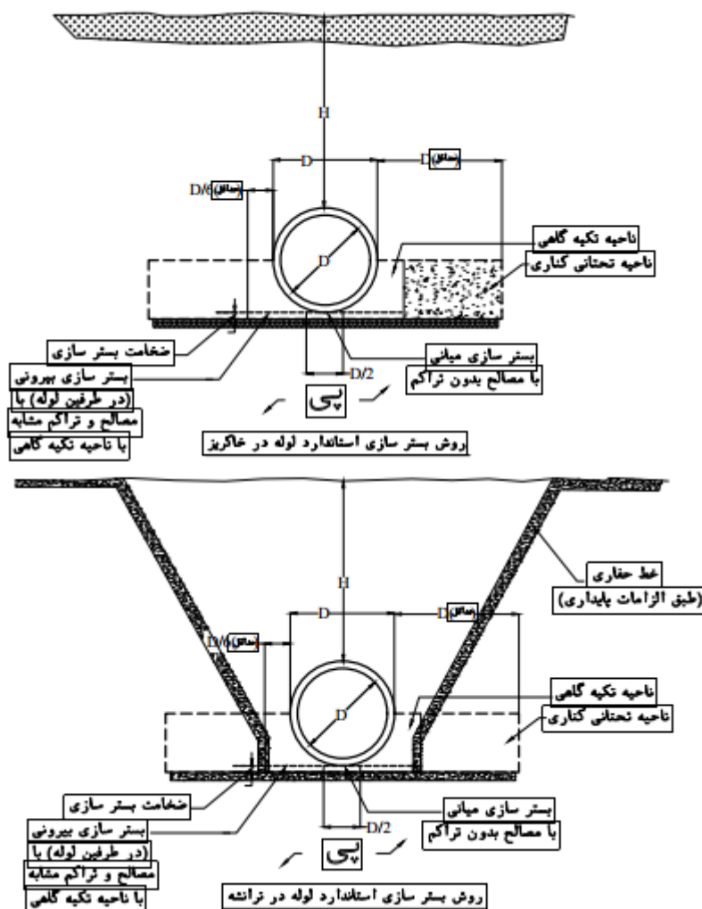
شکل ۴۴: جزئیات اجرایی بستر سازی لوله‌های بتنی
