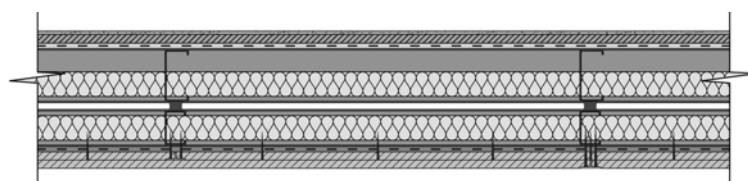
شکل ۴-۲۱- مقطع دیوار خشک دو قابه با وادارهای هم‌راستا
